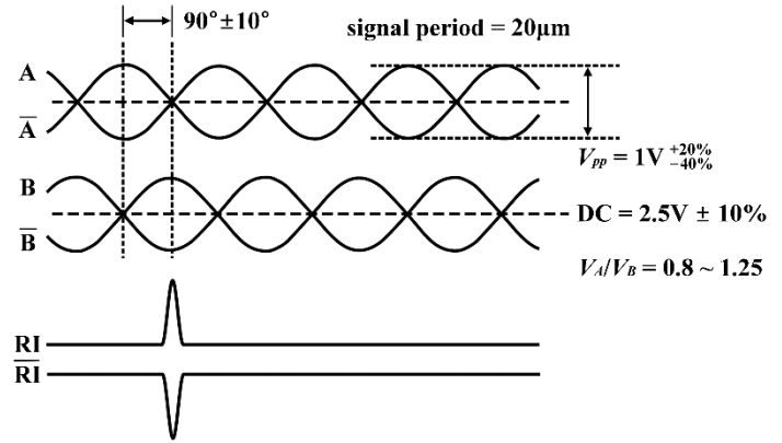
類比式差動弦波 (1 Vpp)
