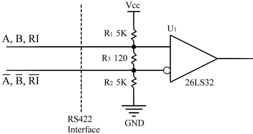
後續計數器參考電路
