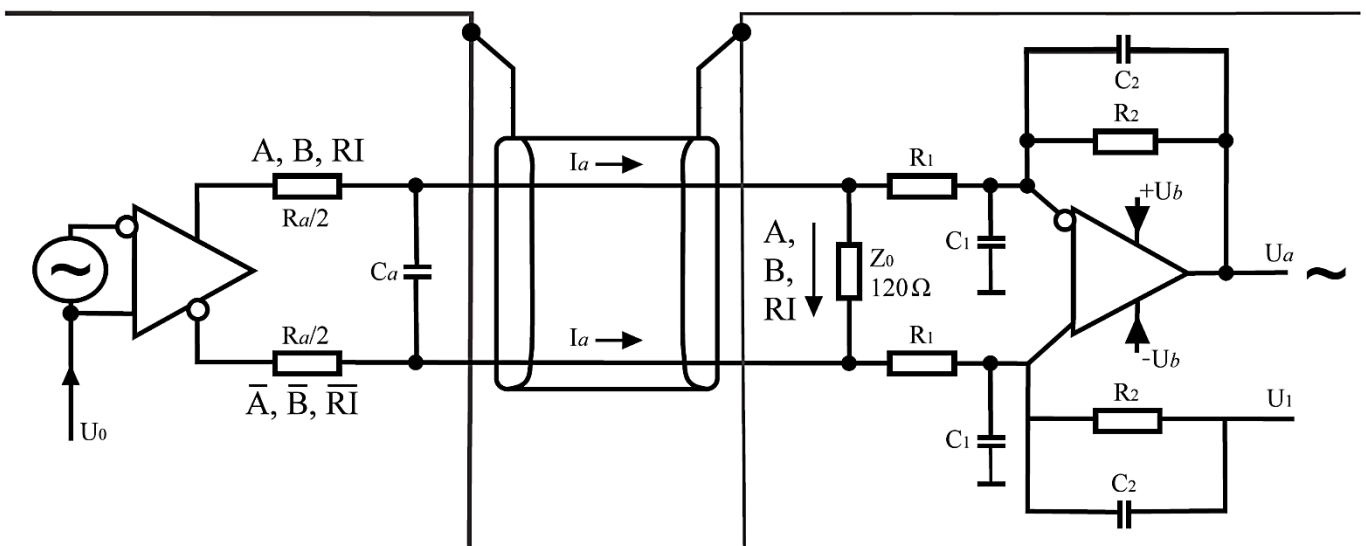
後續介面參考電路
