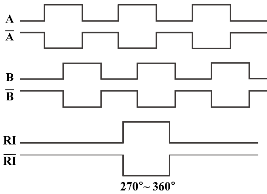
數位式差動方波 (RS422)
